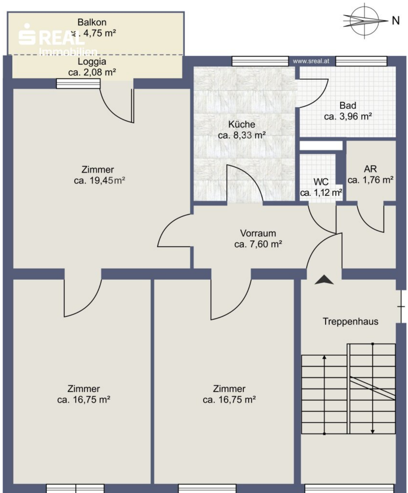
Skizze 4. Obergeschoss
