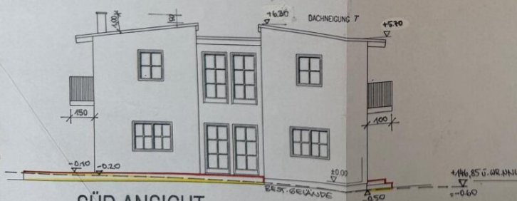
SÜD ANSICHT
