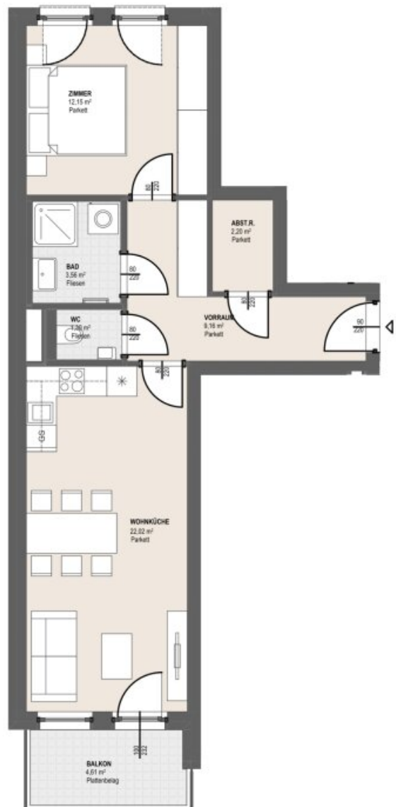
ÜBERSICHT 1. STOCK
