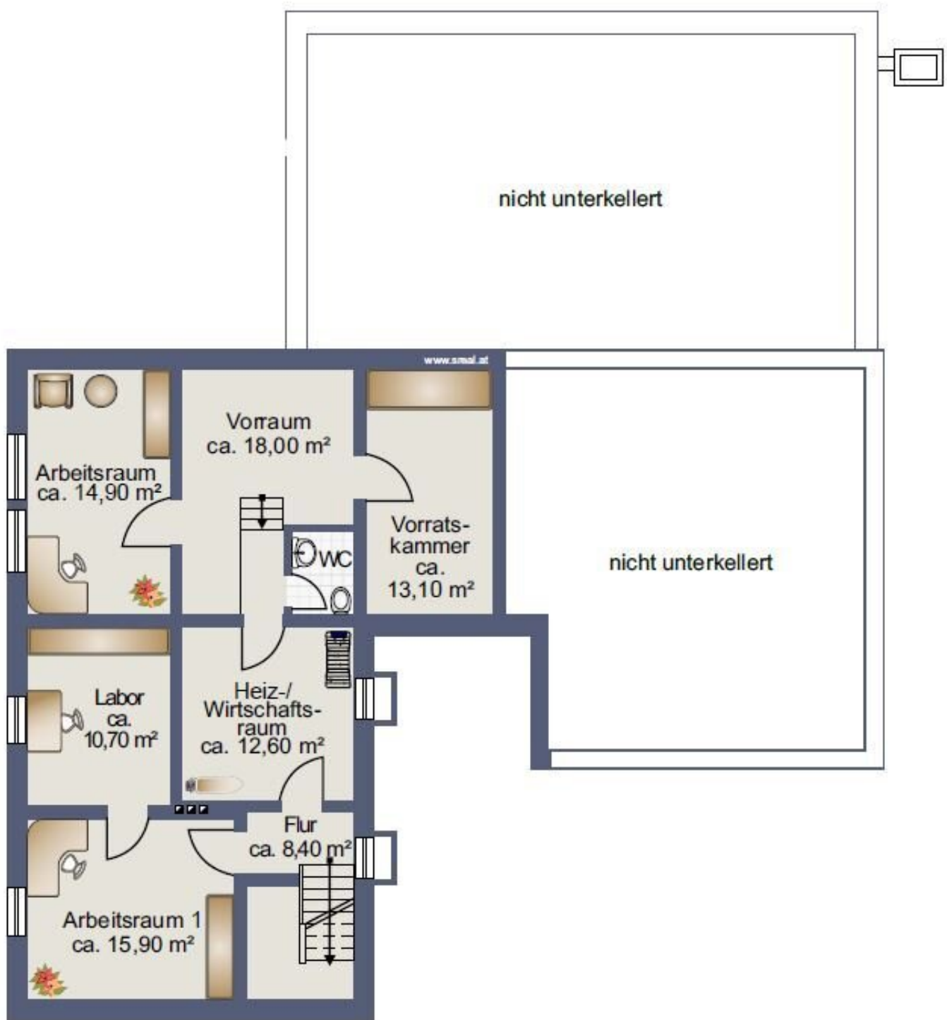
Planskizze Kellergeschoss
