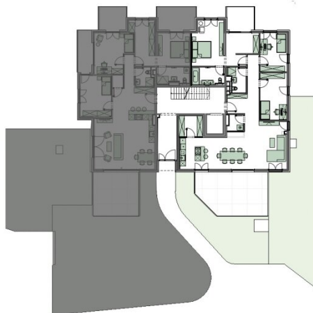
1. Obergeschoß
