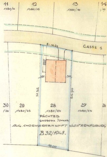
LAGEPLAN 1:500
