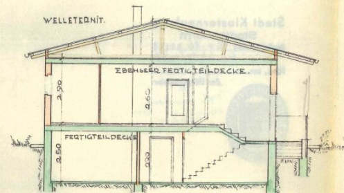
SCHNITT A-B
