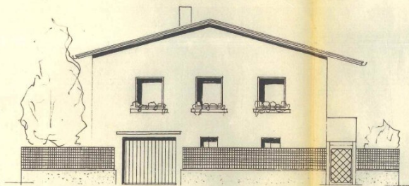
HOBDANSICHT, GASSE
