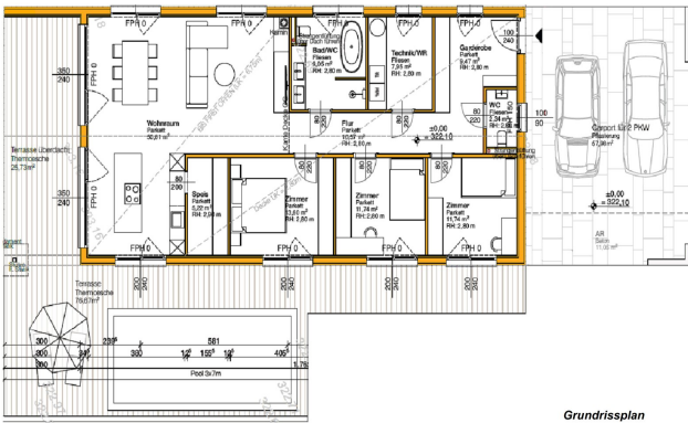
Grundrissplan
