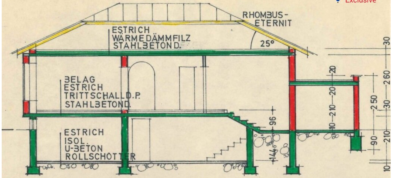
SCHNITT A-B
