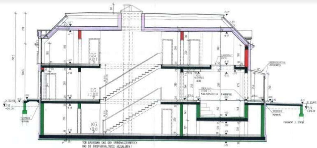
SCHNITT A-A
