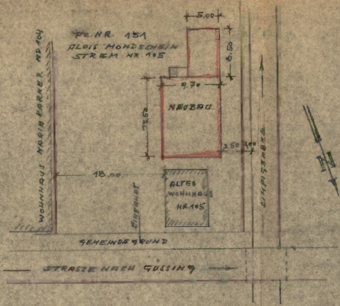
LAGEPLAN 1:500
