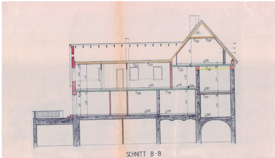
Schnitt
