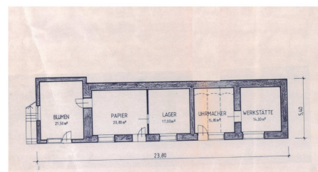
Grundriss Untergeschoss
