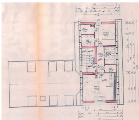
Grundriss Dachgeschoss 1 Einheit
