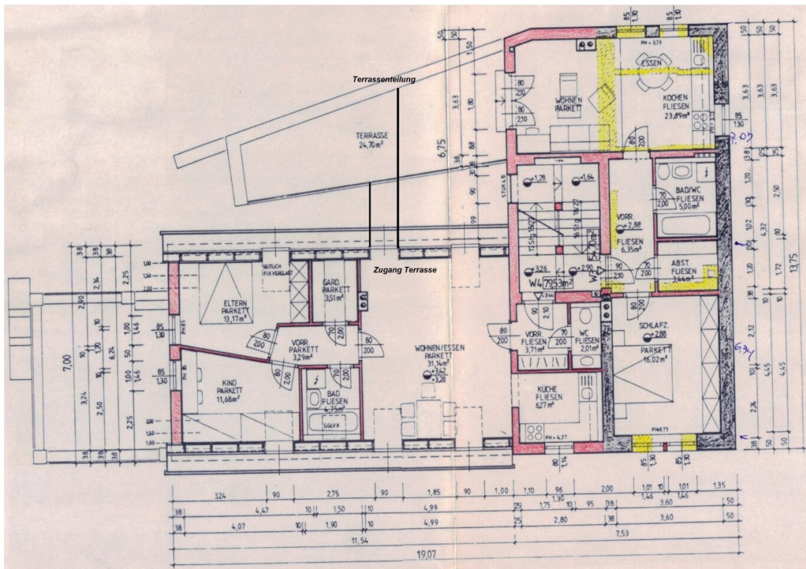
Grundriss Obergeschoss 2 Wohneinheiten
