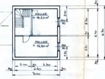
GRUNDRISS Keller
