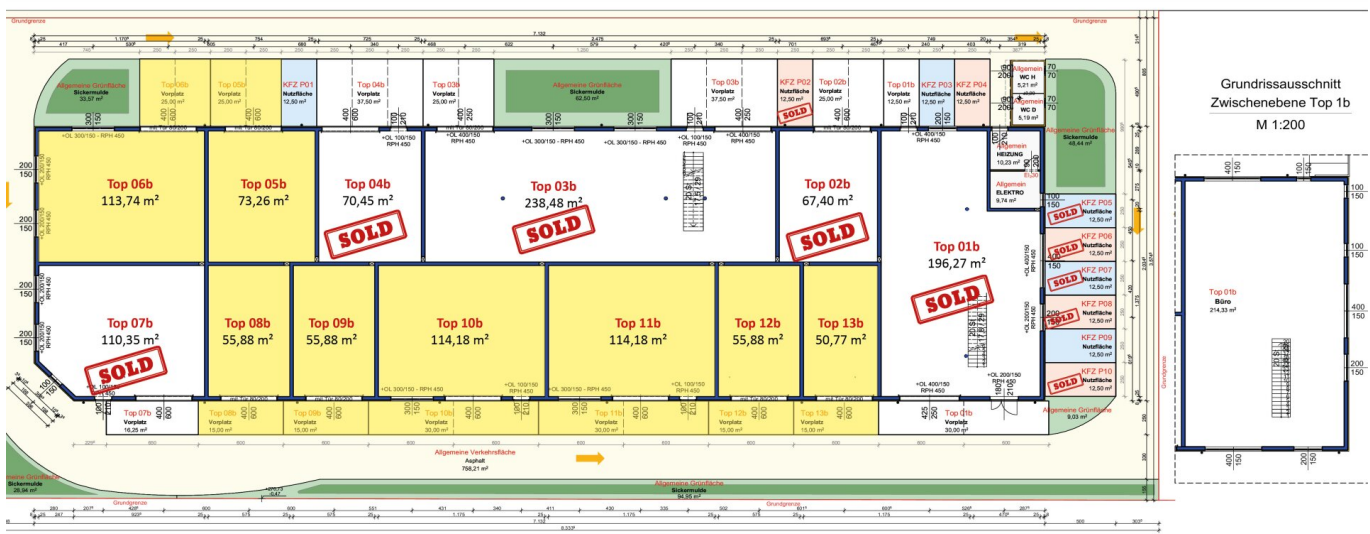
Parfifizierungsplan M 1:200
