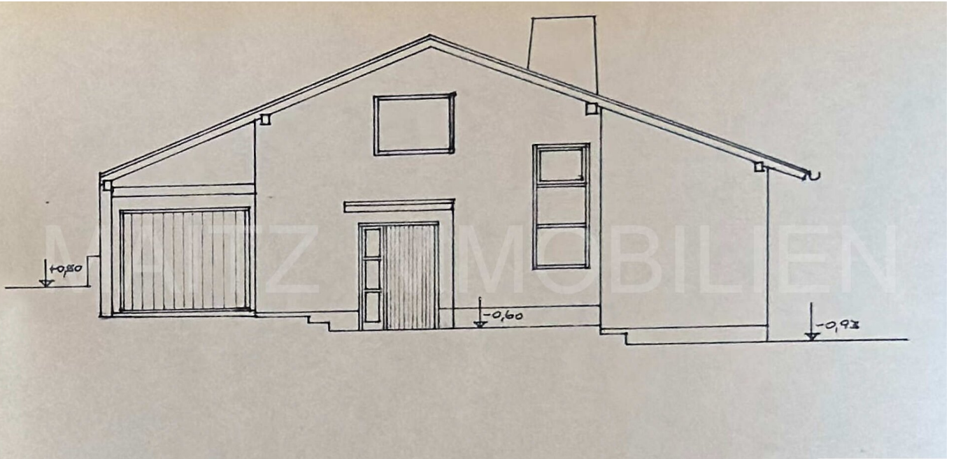
NORDWESTANSICHT 1:100
