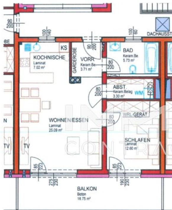
Grundriss Top 6 / Top 7 spiegelsymmetrisch
