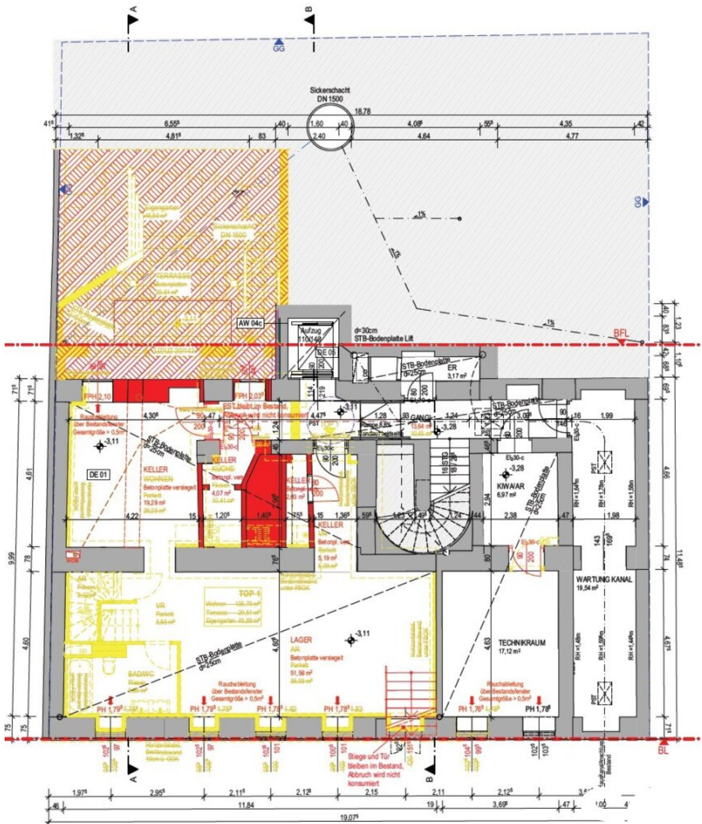
KELLERGESCHOSS
