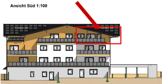
Ansicht Süd 1:100
