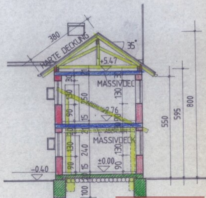
SCHNITT B-B
