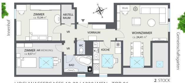
HOCHWASSERGASSE 18-20 | 1230 WIEN - TOP 06 2. STOCK Die im Grundriss abgebildeten Möbel sind nicht inkludiert, sondern nur symbolhaft. Bad & Küche gem. Beschreibungstext möbliert. Der Raum NW seitig mit ca. 9,57 m 2 hat eine Abstellraum-Widmung.
