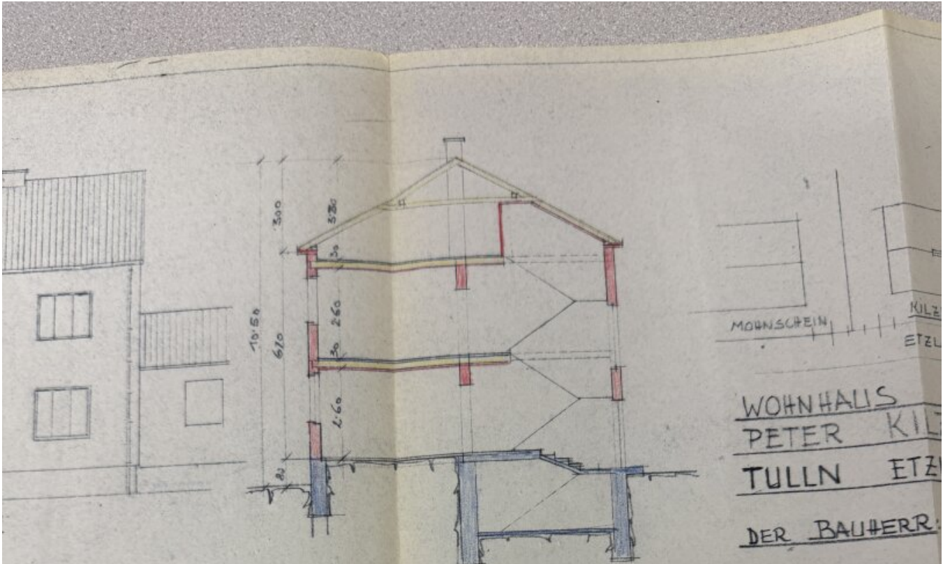
SCHNITT
