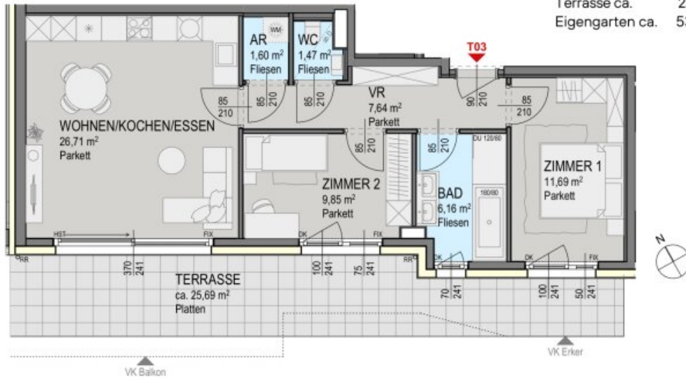
Grundriss Erdgeschoss
