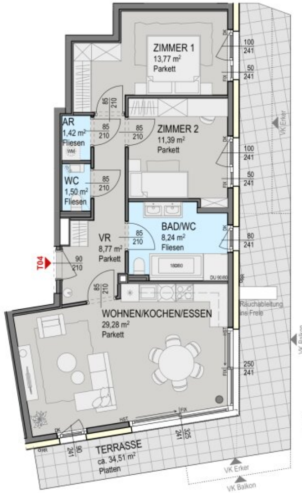
Grundriss Erdgeschoss
