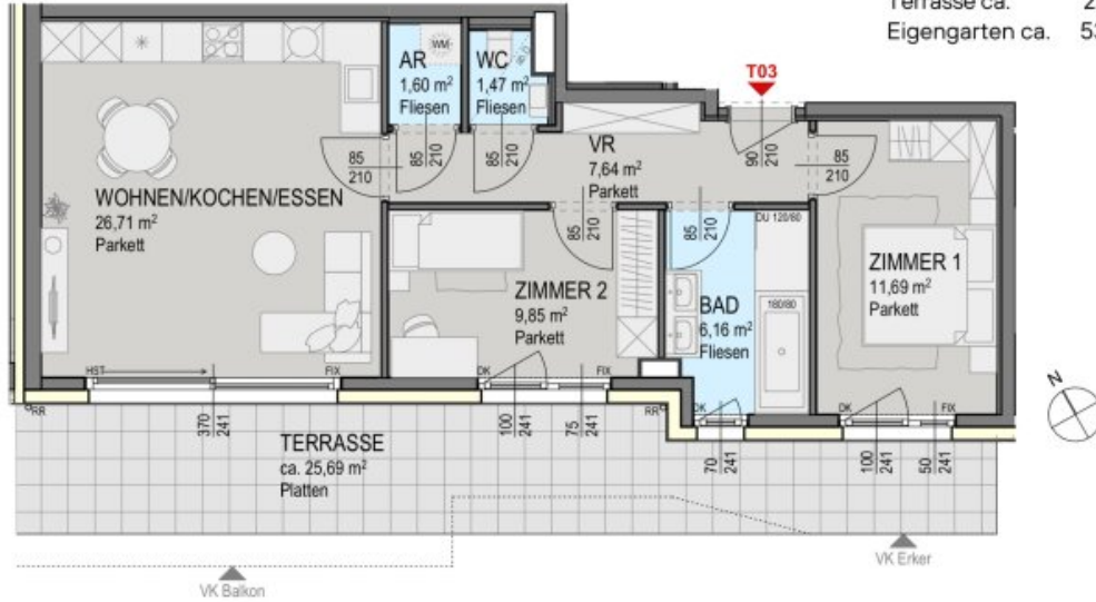
Grundriss Erdgeschoss
