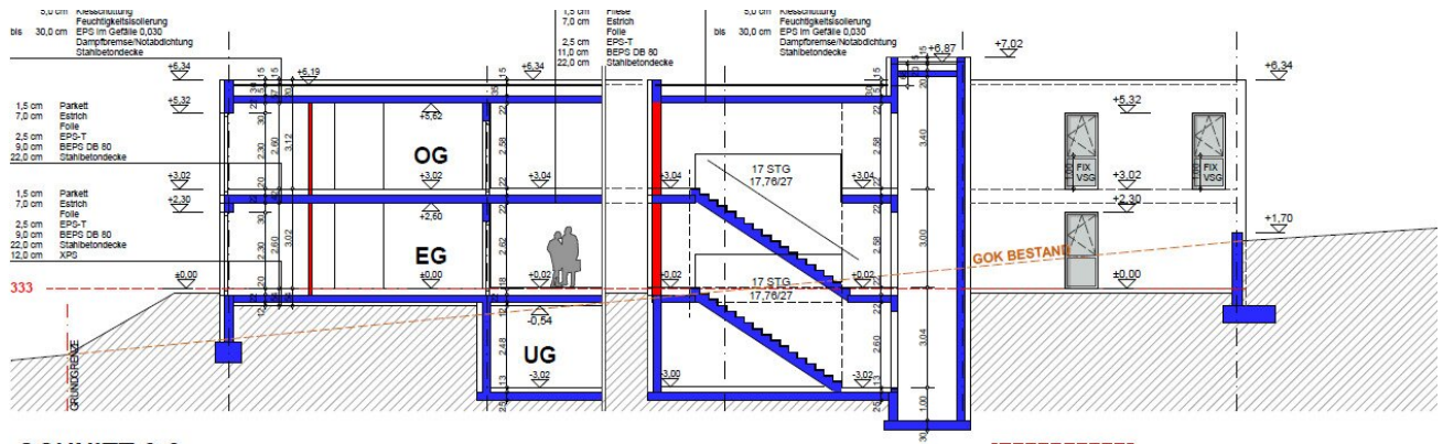
SCHNITT 2-2
