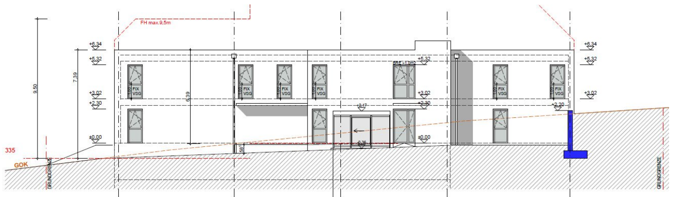
ANSICHT NORDWEST
