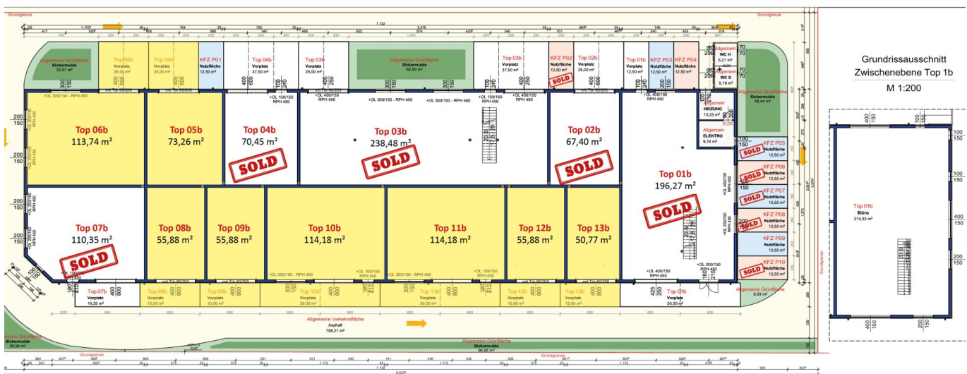
Parfifizierungsplan M 1:200
