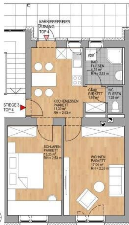
GRUNDRISS 1:100
