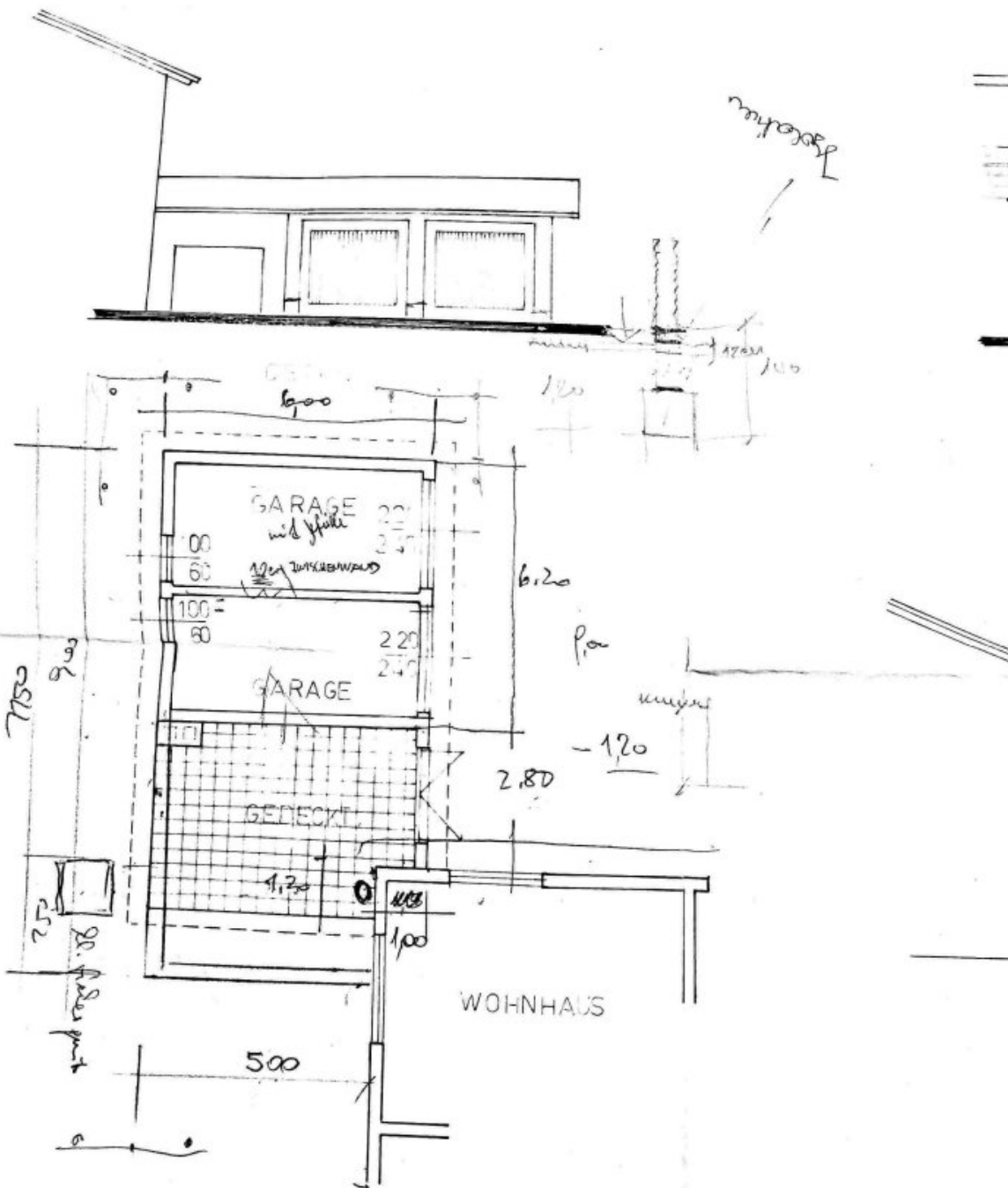
GRUNDRISS
