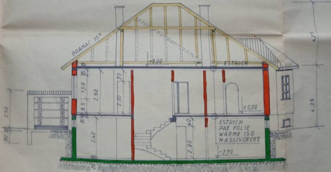
SCHNITT A-B
