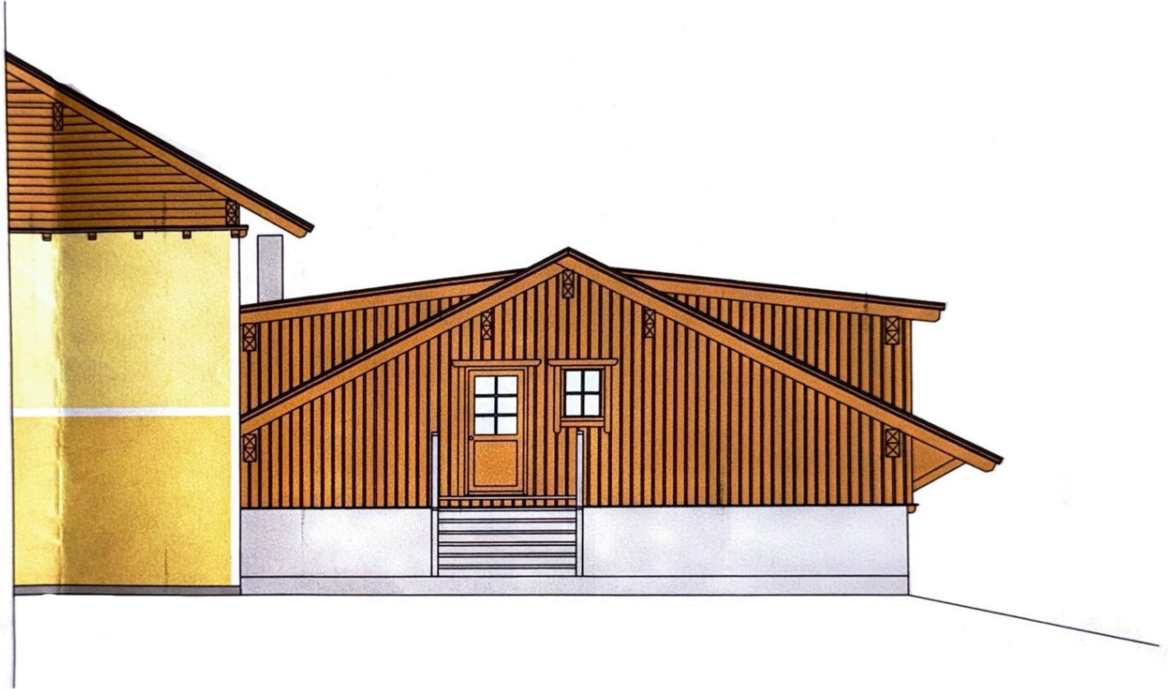
Nordwestansicht
