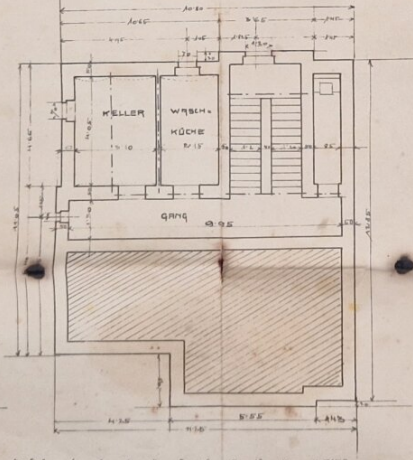
SOUTERRAIN.
