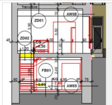
SCHNITT S05:
