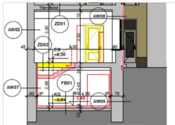
SCHNITT S02:
