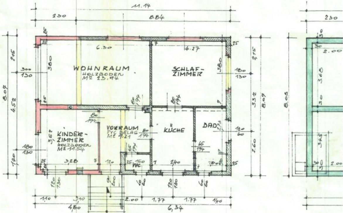
ERDGESCHOSS
