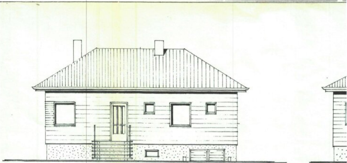
OSTANSICHT
