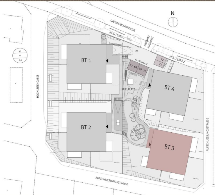
BAUTEIL 1 - 4 LAGEPLAN
