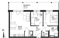
TOP 18 - 2.OG M1100
