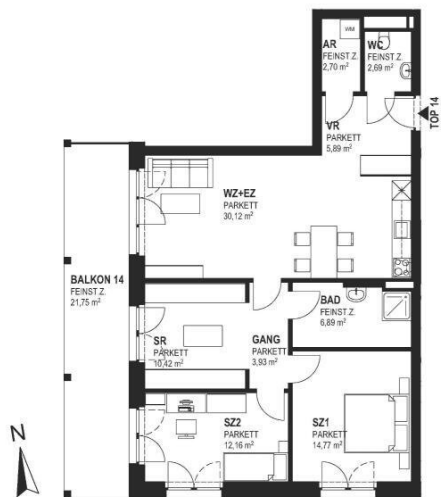
TOP 14 - 1.OG M1:100
