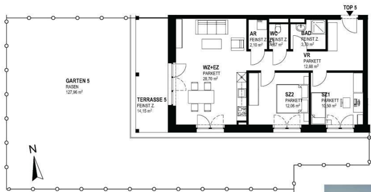
TOP 5 - EG M1:100
