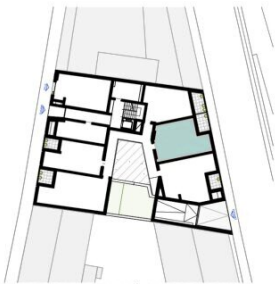
ORIENTIERUNGSPLAN | +0 ERDGESCHOSS
