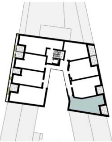
ORIENTIERUNGSPLAN | +1 OBERGESCHOSS
