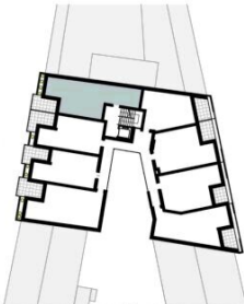
ORIENTIERUNGSPLAN | +2 OBERGESCHOSS
