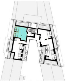
ORIENTIERUNGSPLAN | +6 DACHGESCHOSS 02
