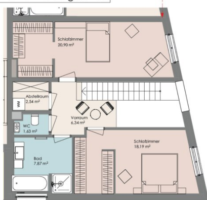
GRUNDRISS TOP M2 - Obergeschoss
