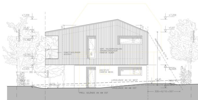
ANSICHT OST | M 1/100
