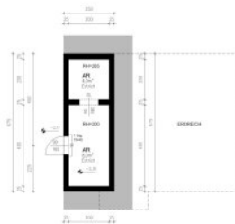
GR UNTERGESCHOSS | M 1:100
