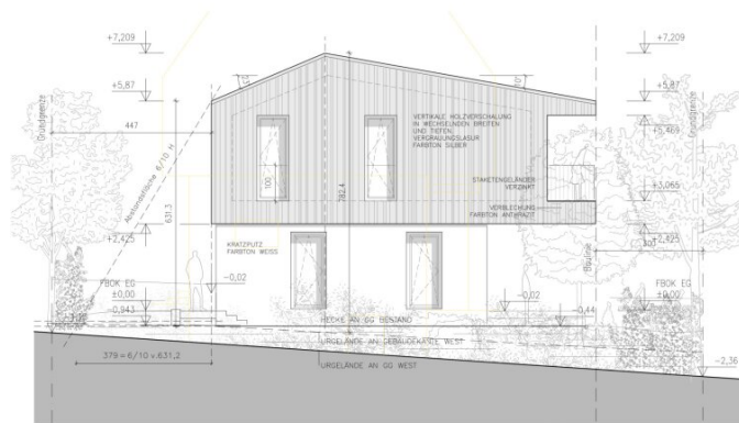
ANSICHT WEST | M 1/100
