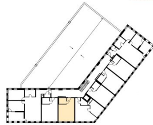
Geschossübersicht
