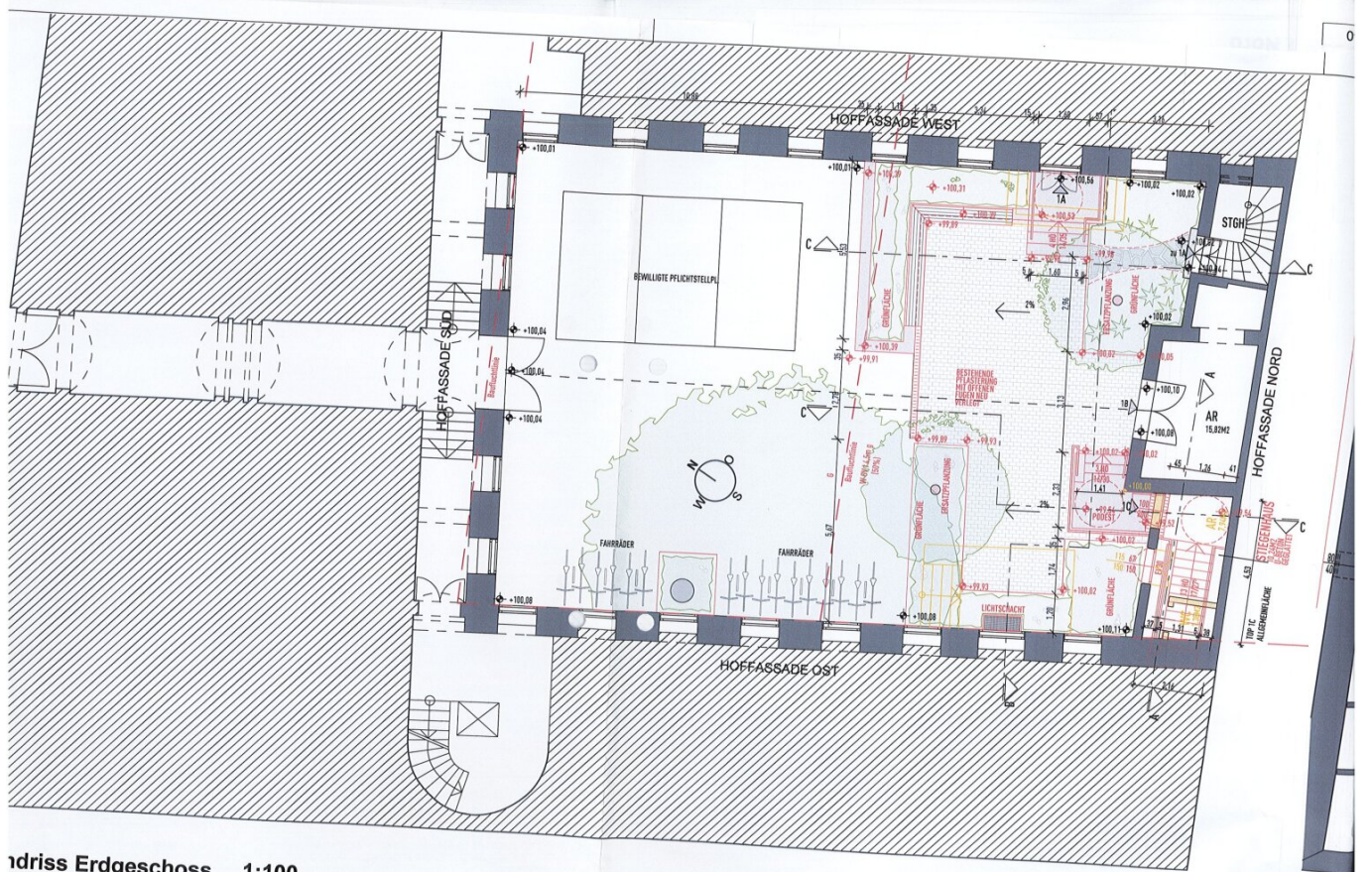
ndriss Erdgeschoss 1:100
