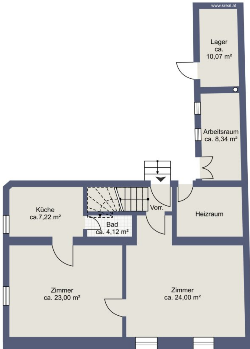
Skizze Erdgeschoss
