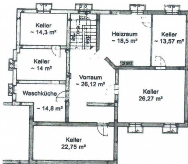
Kellergeschoß
