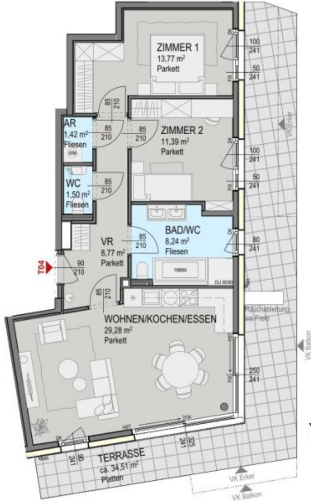
Grundriss Erdgeschoss
