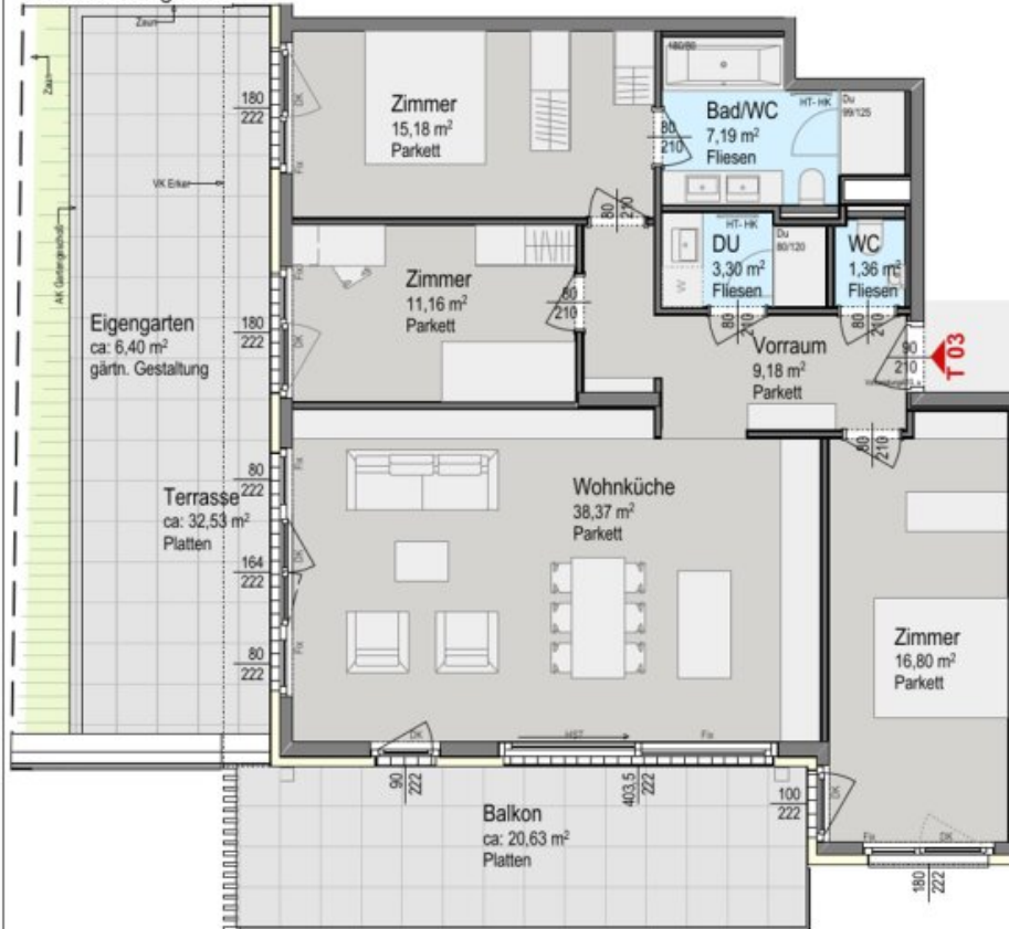
Grundriss Erdgeschoß
