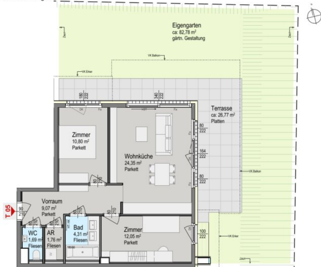
Grundriss Erdgeschoß
