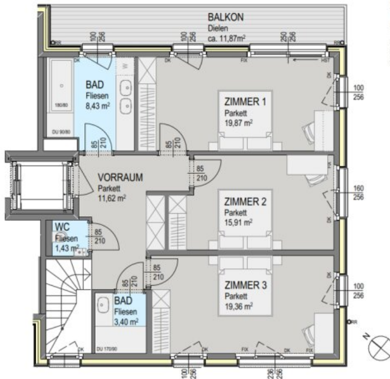
Grundriss Obergeschoss
